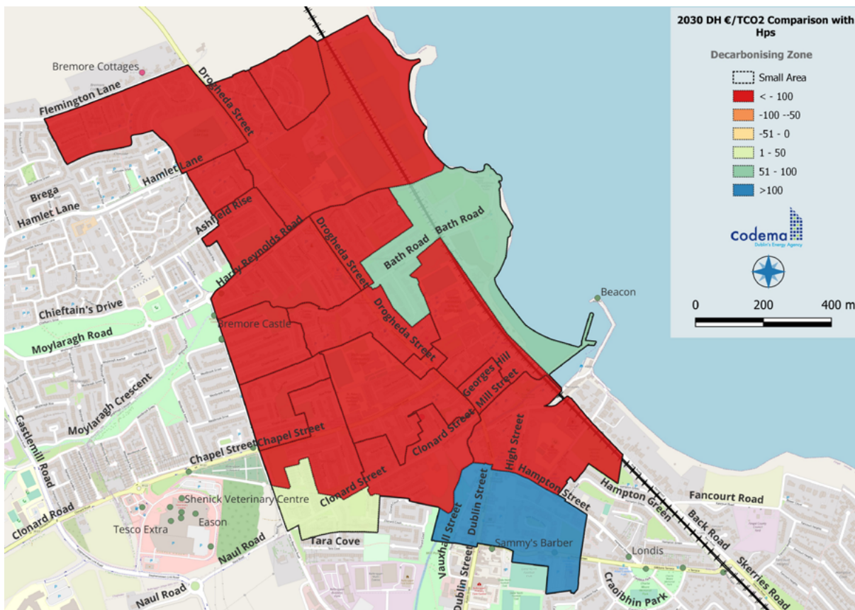
Fíor 6.15: Teaschaidéil agus poitéinseal oiriúnachta téimh ceantair i gCD Bhaile Brigín
