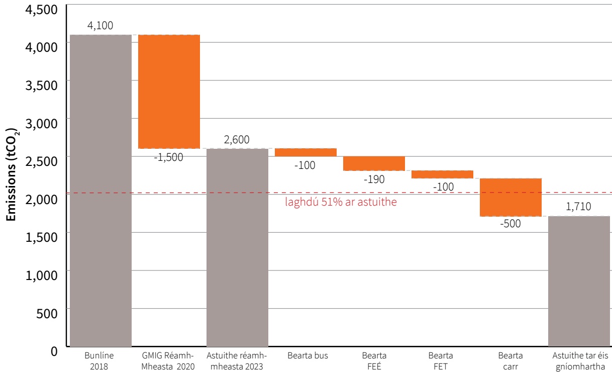
Fíor 6.12: Conair Aeráide Iompair CD Bhaile Brigín
