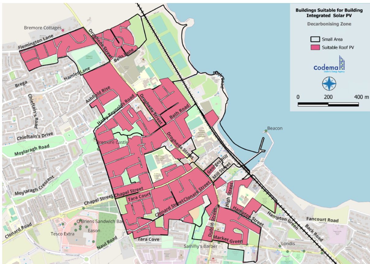
Fíor 6.13: Deis fhéideartha leictreachais gréine ar bharr an dín i gCD Bhaile Brigín
