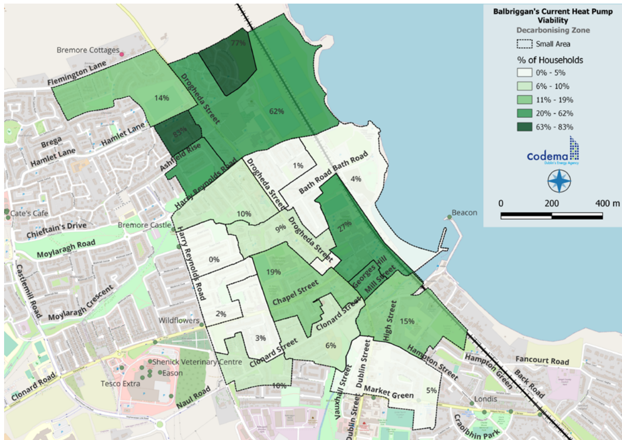
Fíor 6.14: Acmhainn oiriúnachta teaschaidéil i gCD Bhaile Brígin
